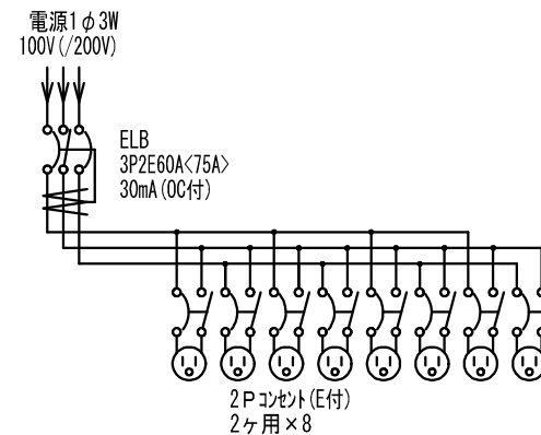
結線図
